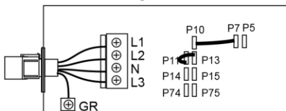
Trefasanslutning med enkel neutral
