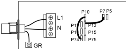
Enfasanslutning
