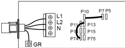
Tvåfasanslutning
