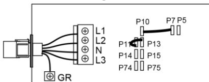
Trefasanslutning med enkel neutral
