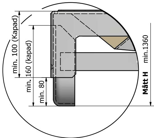
Detalj X med max mått
