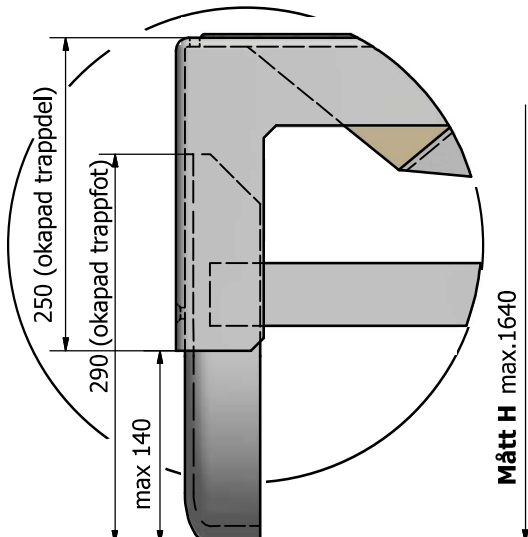
Detalj X med max mått
