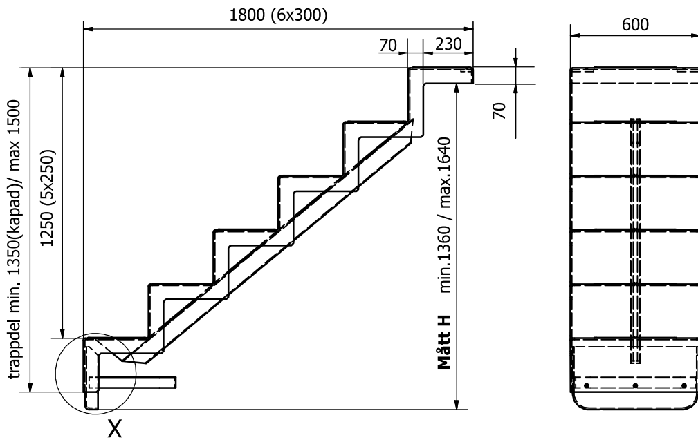
Detalj X med min mått
