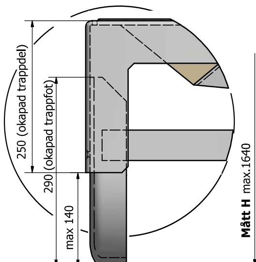
Detalj X med max mått
