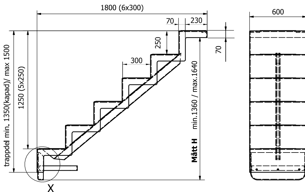
Detalj X med min mått
