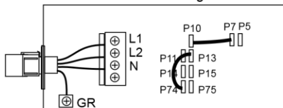
Tvåfasanslutning
