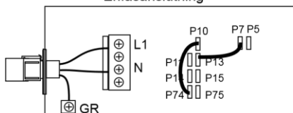
Enfasanslutning
